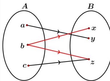
(b) Contoh Bukan Fungsi
