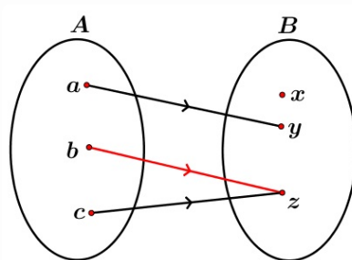
(a) Contoh Fungsi
